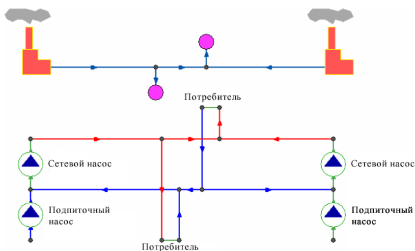
Рисунок 2.2. Сверху: однолинейное изображение сети, снизу – внутренне представление
