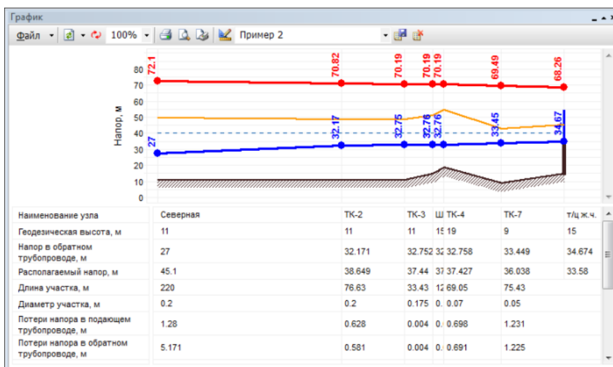
Рисунок 17.13. Пример автоматического масштаба графика
