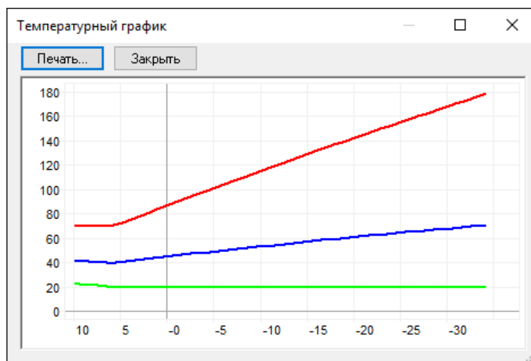
Рисунок 13.6. Температурный график в результате расчета
