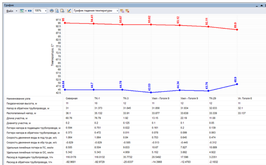
Рисунок 1.3. График падения температуры
