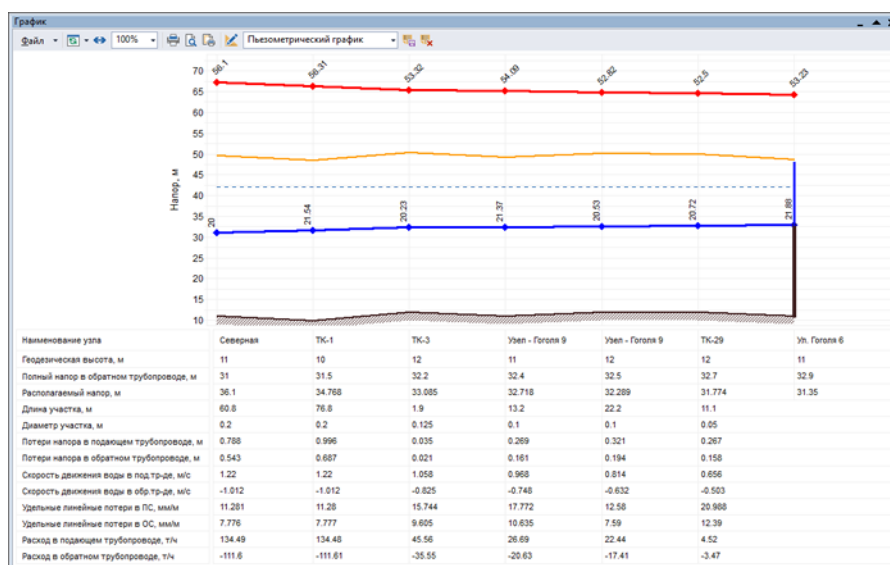
Рисунок 1.2. Пример пьезометрического графика
