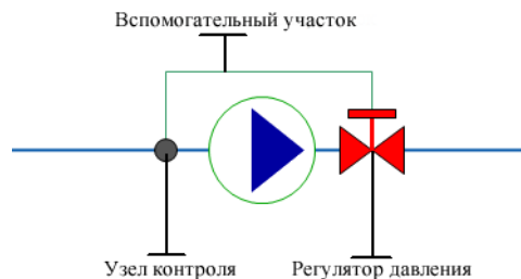
Рисунок 2.38. Регулятор давления «до себя» на подающем трубопроводе
