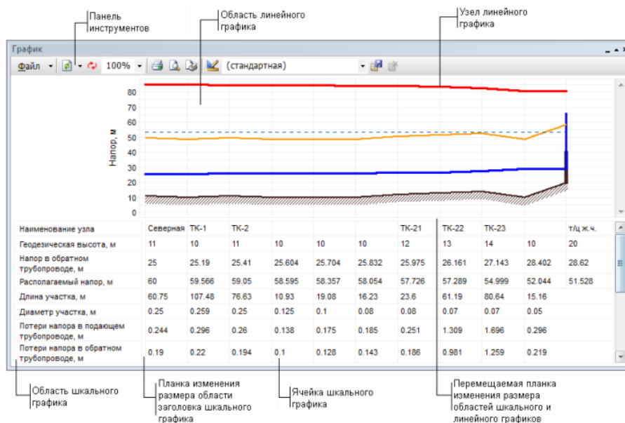
Рисунок 17.3. Окно пьезометрического графика
