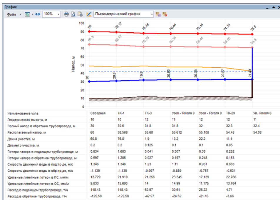
Рисунок 17.8. Совмещение пьезометрических графиков
