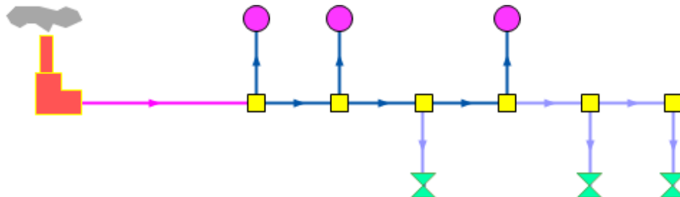
Рисунок 2.26. Пример тепловой сети, работающей на слив
