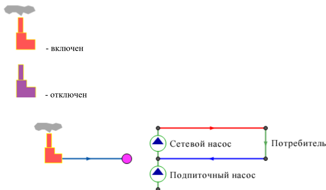
Рисунок 2.1. Слева однолинейное изображение сети, справа – внутреннее представление
