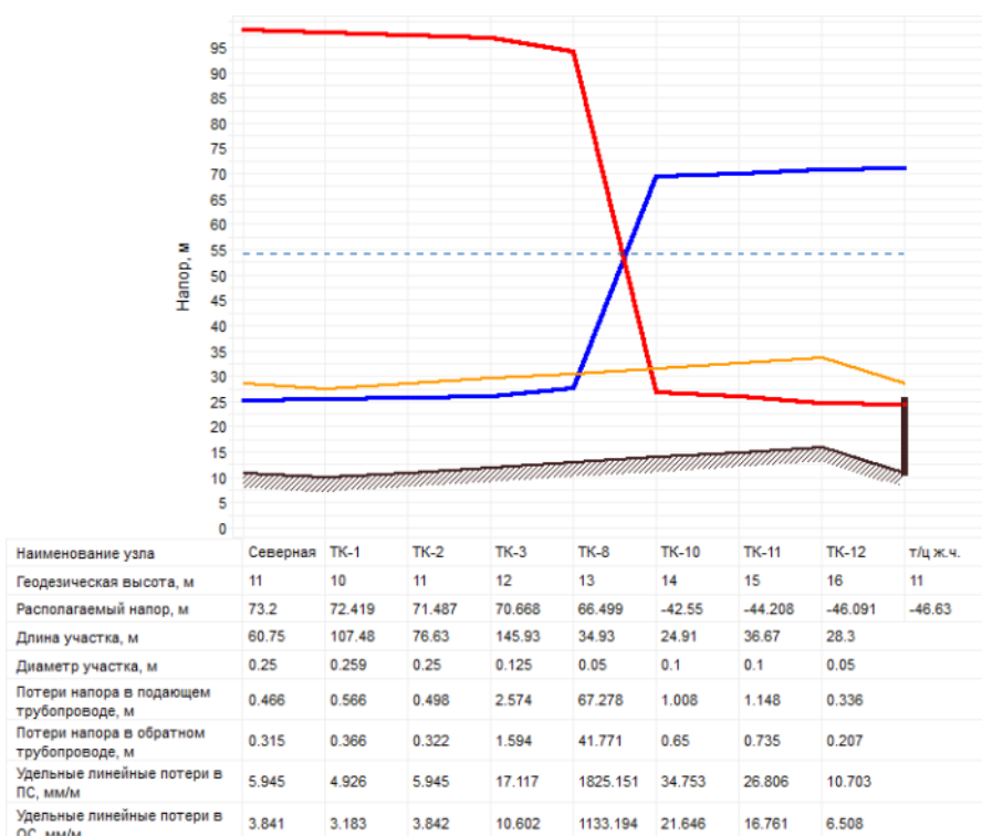
Рисунок 18.7. Обнаружение ошибки с помощью пьезометрического графика
