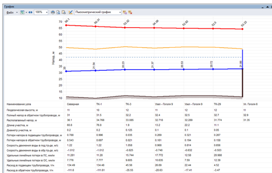
Рисунок 17.4. Пример пьезометрического графика
