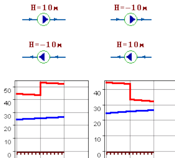
Рисунок 2.21. Моделирование работы насоса напором
