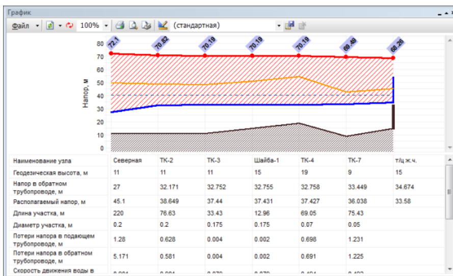
Рисунок 17.25. Пример графика с надписями
