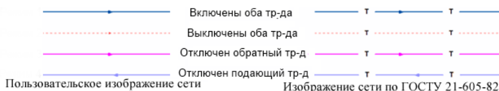
Рисунок 2.4. Режимы изображения участка
