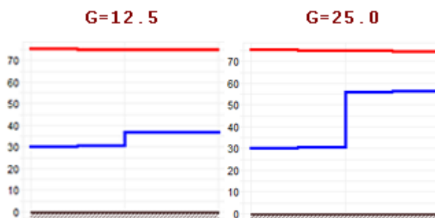
Рисунок 2.36. Локальное сопротивление на обратном трубопроводе
