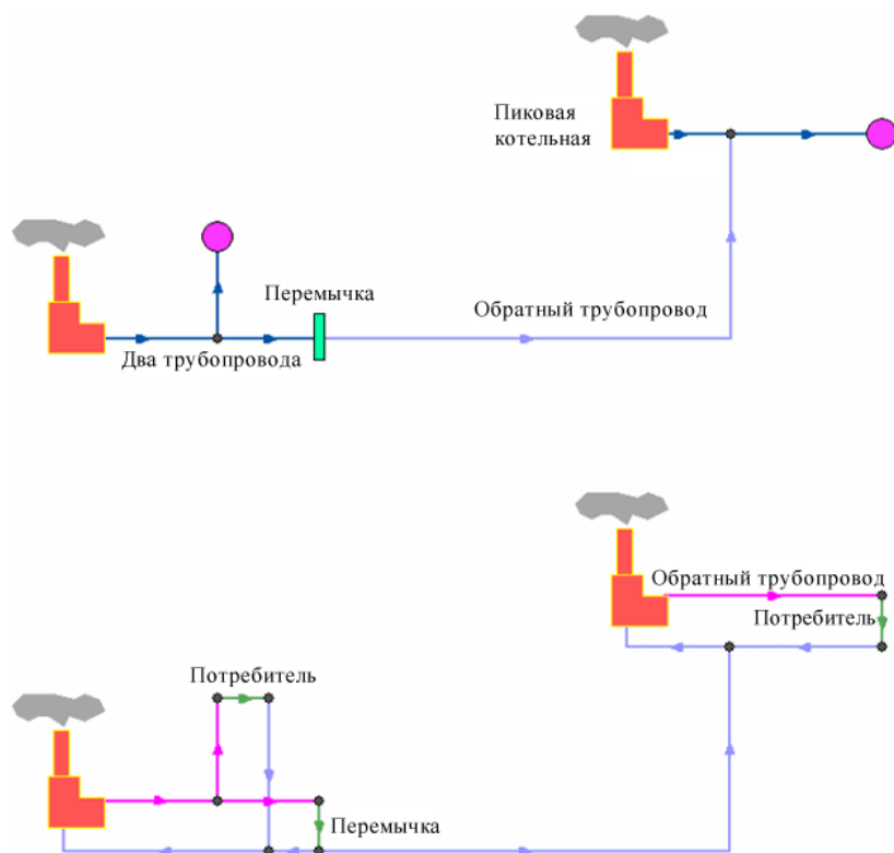
Рисунок 2.3. Сверху: однолинейное изображение сети, снизу – внутренне представление
