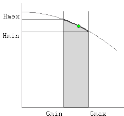
Рисунок 2.22. Моделирование работы насоса QH характеристикой
